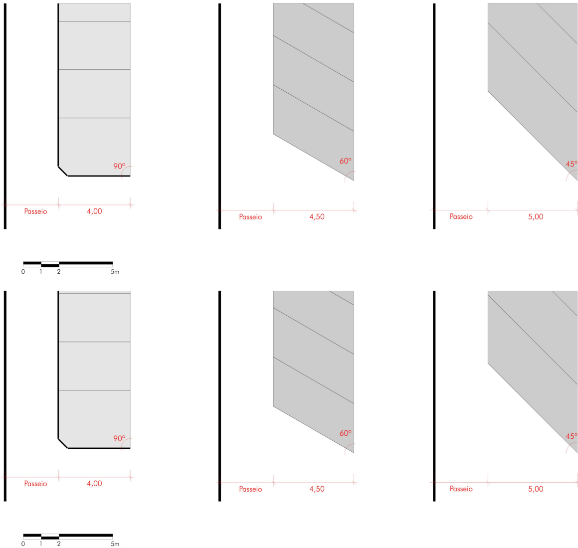
FIGURA 2: LARGURAS MÍNIMAS DE FAIXAS DE ESTACIONAMENTO.
